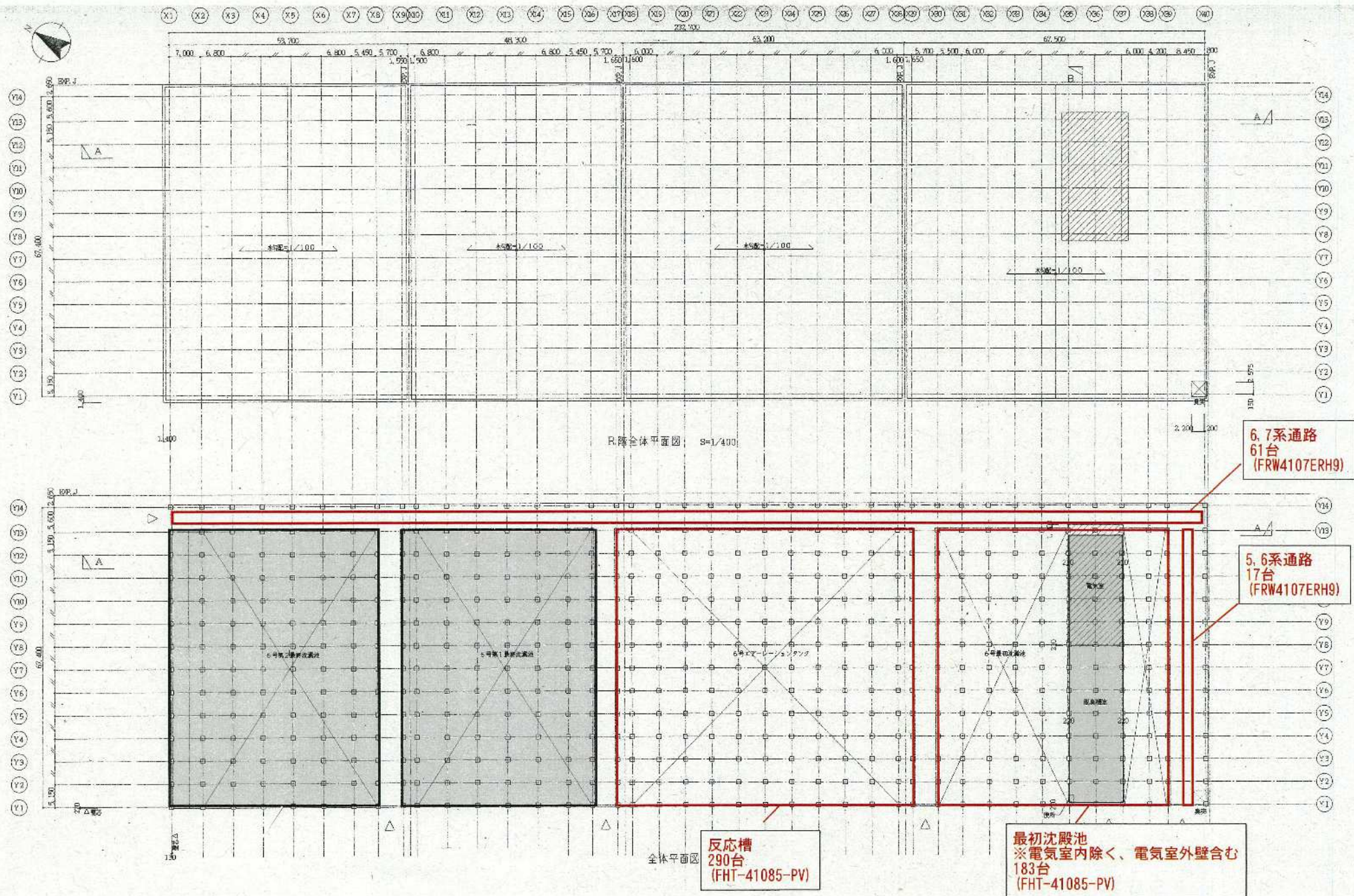
図面名 6系水処理最初沈殿池・反応槽平面図 図番 2
